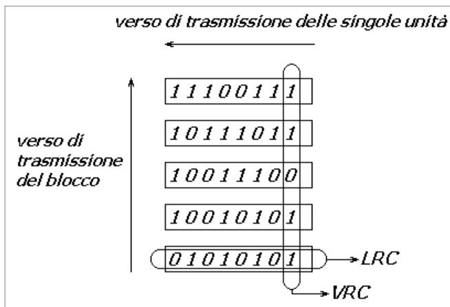
Figura 22: Algoritmo LRC.
